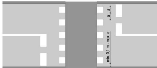
Slika 45. Okomiti prijelaz biciklističke staze ili biciklističke trake preko kolnika
