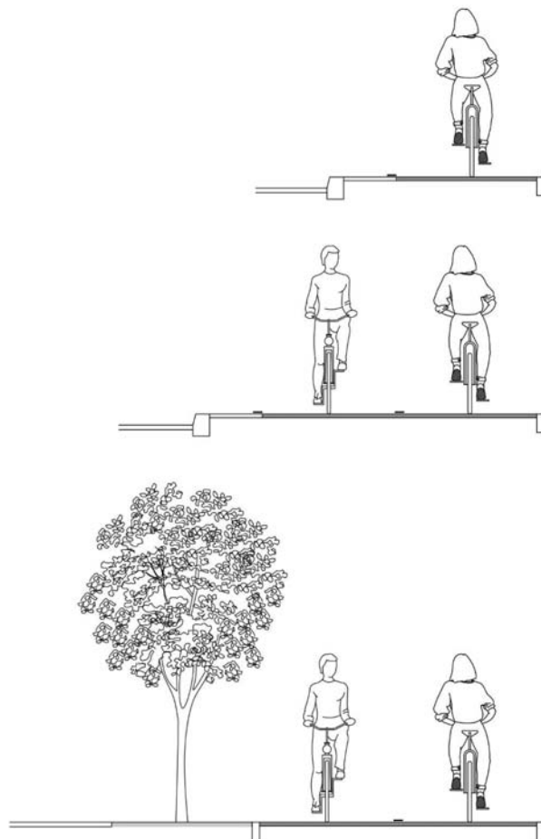
Slika 2. Vrste biciklističkih staza
