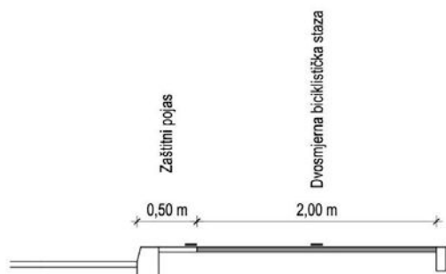
Slika 10. Dimenzije dvosmjerne biciklističke staze u naselju
