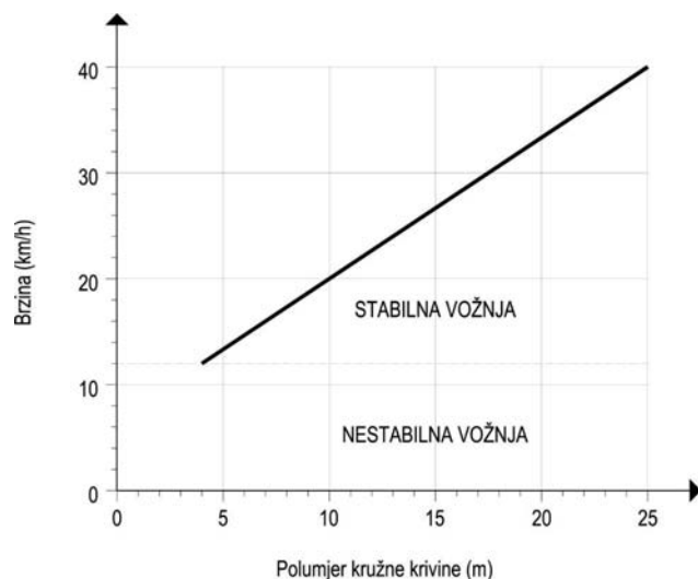
Slika 18. Dijagram odnosa projektne brzine i veličine polumjera kružne krivine
