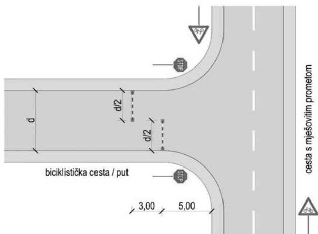
Slika 40. Spoj biciklističke ceste/puta s cestom za mješoviti promet
