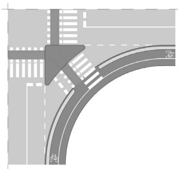
Slika 26: Zajedničko vođenje biciklističkog i pješačkog prometa preko razdjelnih otoka
