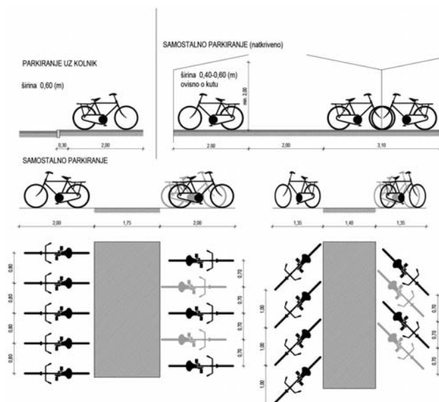
Slika 50. Standardne dimenzije parkirališnih mjesta za bicikle
