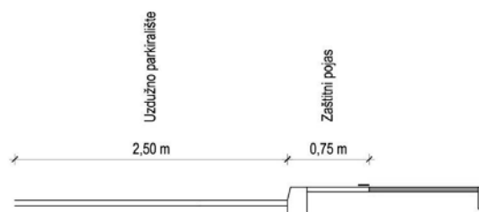
Slika 12. Zaštitni pojas biciklističke staze uz trak za uzdužno parkiranje
