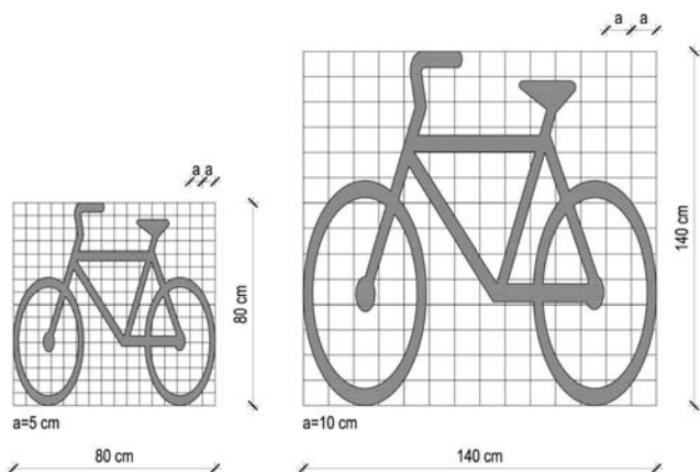
Slika 48. Piktogram bicikla
