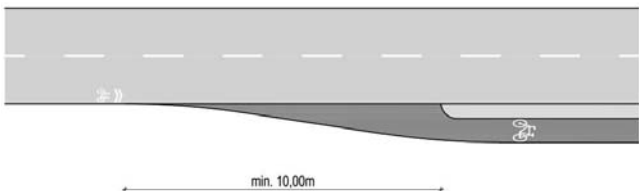
Slika 34. Tehničko rješenje prijelaza biciklista s kolnika na biciklističku stazu
