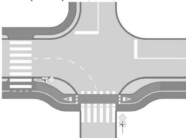
Slika 24. Vođenje biciklističkog prometa preko privoza ceste s prednošću prolaska
