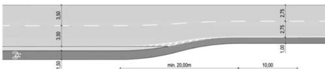
Slika 32. Tehničko rješenje prijelaza biciklističke staze na biciklističku traku
