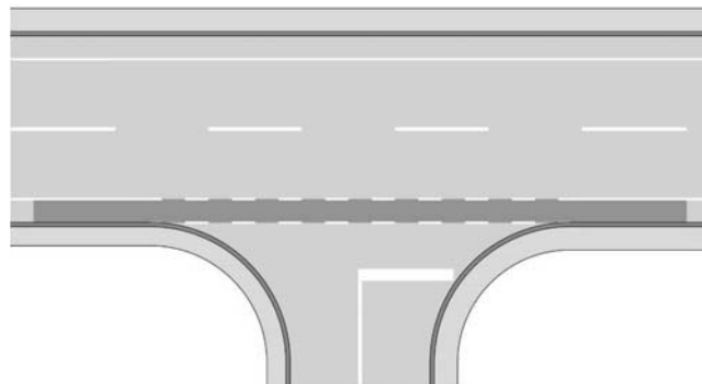
Slika 21. Izravno vođenje biciklističke trake preko privoza sporedne ceste
