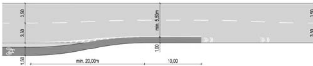
Slika 33. Tehničko rješenje prijelaza biciklističke staze na kolnik s mješovitim prometom
