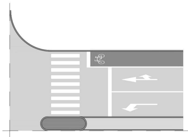
Slika 30. Pomaknuta crta zaustavljanja za bicikliste
