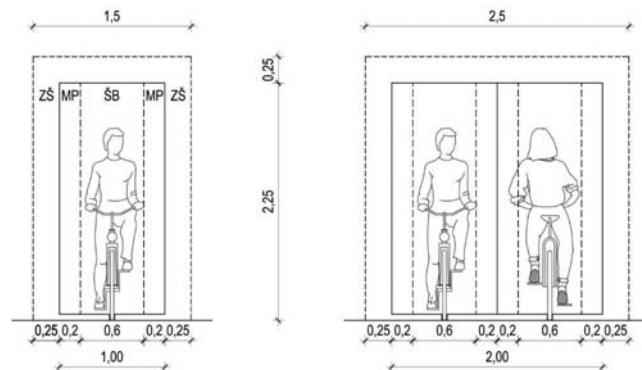
Slika 6. Slobodni i prometni profil za promet jednog i dva biciklista
