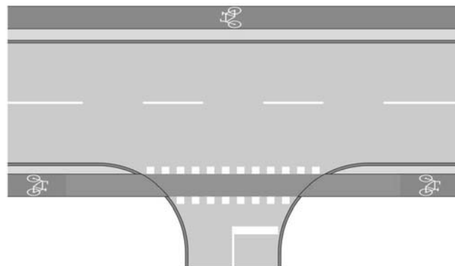
Slika 22. Izravno vođenje biciklističke staze preko privoza sporedne ceste
