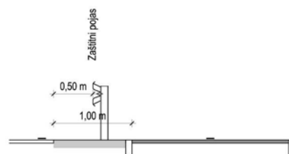
Slika 14. Zaštitni pojas biciklističke staze uz cestu izvan naselja sa zaštitnom ogradom
