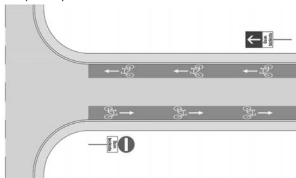
Slika 39. Izvedba obostranih biciklističkih traka u jednosmjernoj ulici
