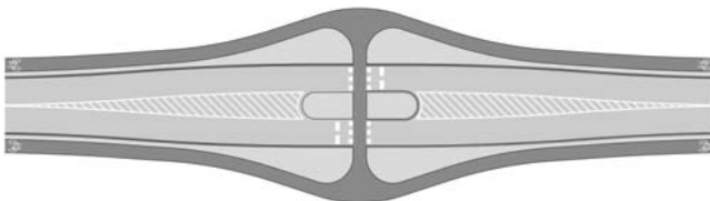
Slika 29. Križanje biciklističkog i motornog prometa izvan zone raskrižja
