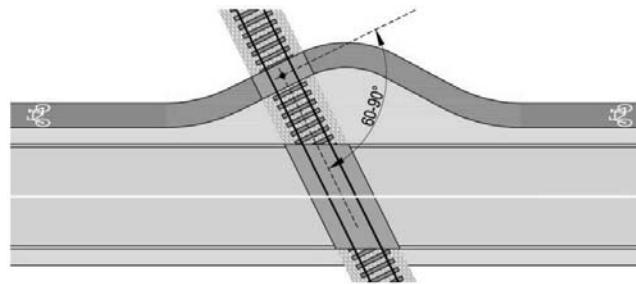
Slika 43. Prijelaz biciklističke prometnice preko željezničke pruge
