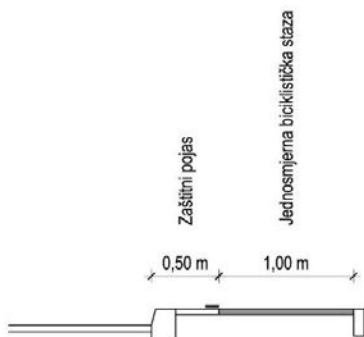
Slika 9. Dimenzije jednosmjerne biciklističke staze u naselju
