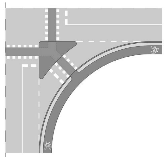
Slika 25: Vođenje biciklističkog prometa preko razdjelnih otoka
