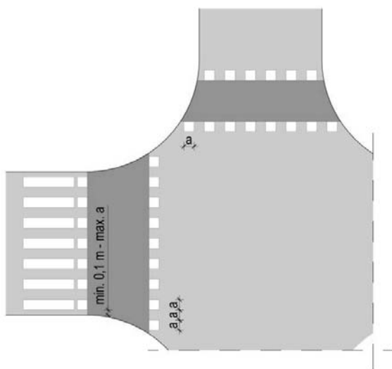
Slika 44. Prijelaz biciklističke staze ili biciklističke trake preko raskrižja
