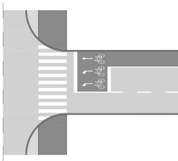
Slika 31. Pomaknuta crta zaustavljanja za biciklista sa površinom za zaustavljanje biciklista
