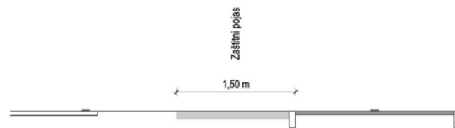
Slika 13. Zaštitni pojas biciklističke staze uz cestu izvan naselja bez zaštitne ograde
