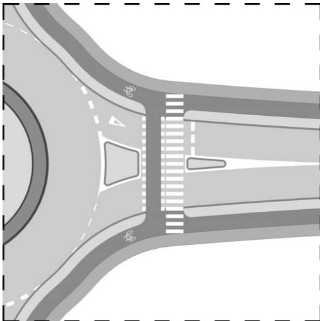
Slika 28. Prijelaz biciklističke staze preko kraka raskrižja s kružnim tokom prometa
