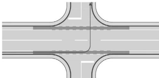
Slika 19. Način lijevog skretanja biciklista u raskrižju s biciklističkom trakom
