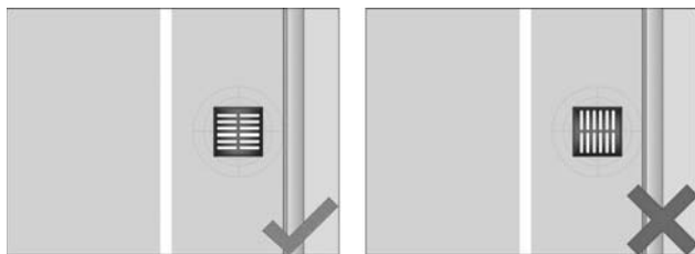
Slika 41. Pravilno i nepravilno usmjerene rešetke na odvodnim šahtovima
