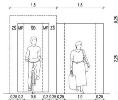
Slika 7. Slobodni i prometni profil za promet jednog biciklista i pješaka
