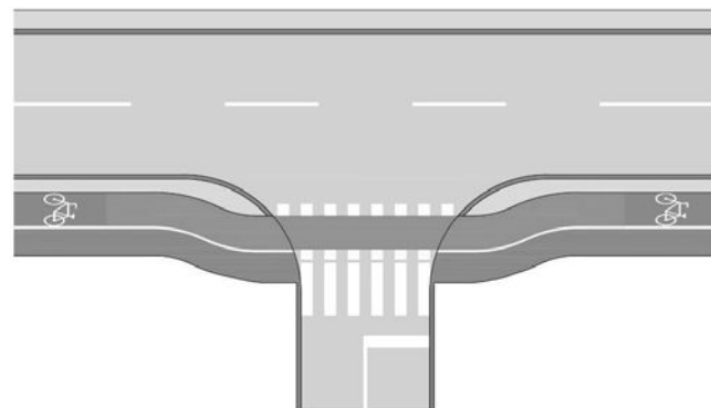
Slika 23. Izmaknuto vođenje biciklističke staze preko privoza sporedne ceste
