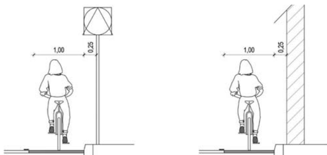
Slika 15. Širina zaštitnog pojasa biciklističke trake uz stalne prepreke
