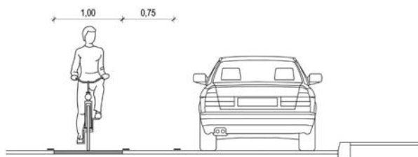
Slika 16. Širina zaštitnog pojasa biciklističke trake uz trak uzdužno parkiranje
