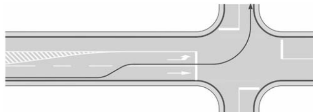
Slika 20. Način lijevog skretanje bicikliste u raskrižju ceste za mješoviti promet
